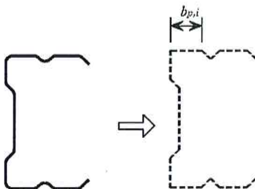
б) идеализированное поперечное сечение
