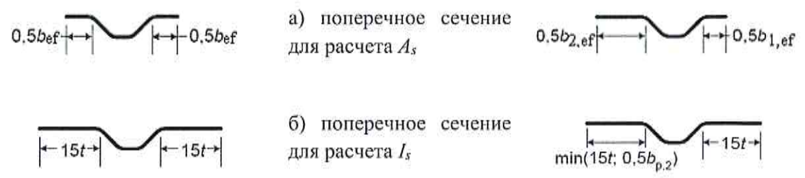
Рисунок 7.10 – Включение в ребро жесткости примыкающих участков полки
